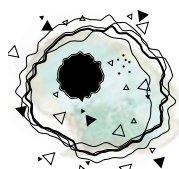
I radicali liberi attaccano la cellula
