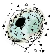
Cellula colpita da stress ossidativo
